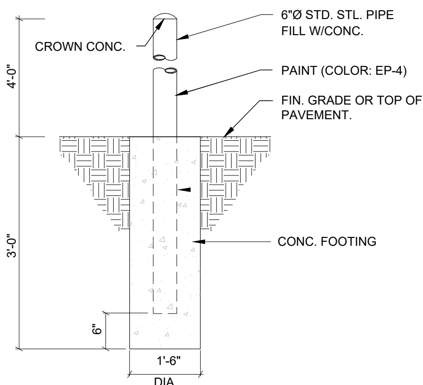
14 BOLLARD DETAIL AS2.3 SCALE: 3/8" = 1'-0"
