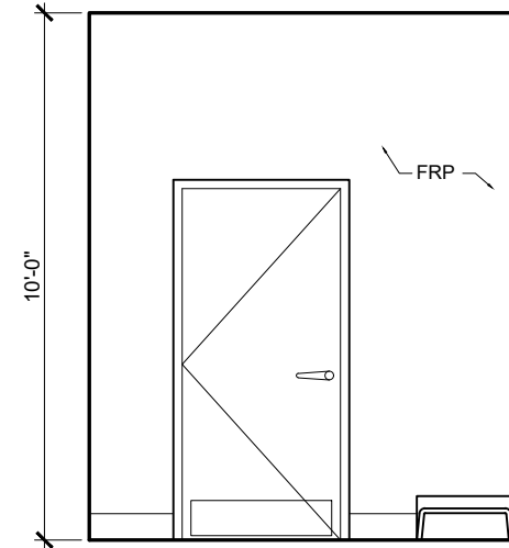
8 WET AREA A9.1 SCALE: 1/4" = 1'-0"
