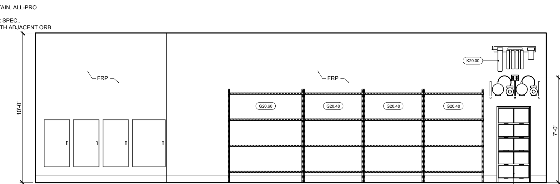
6 WET AREA A9.1 SCALE: 1/4" = 1'-0"
