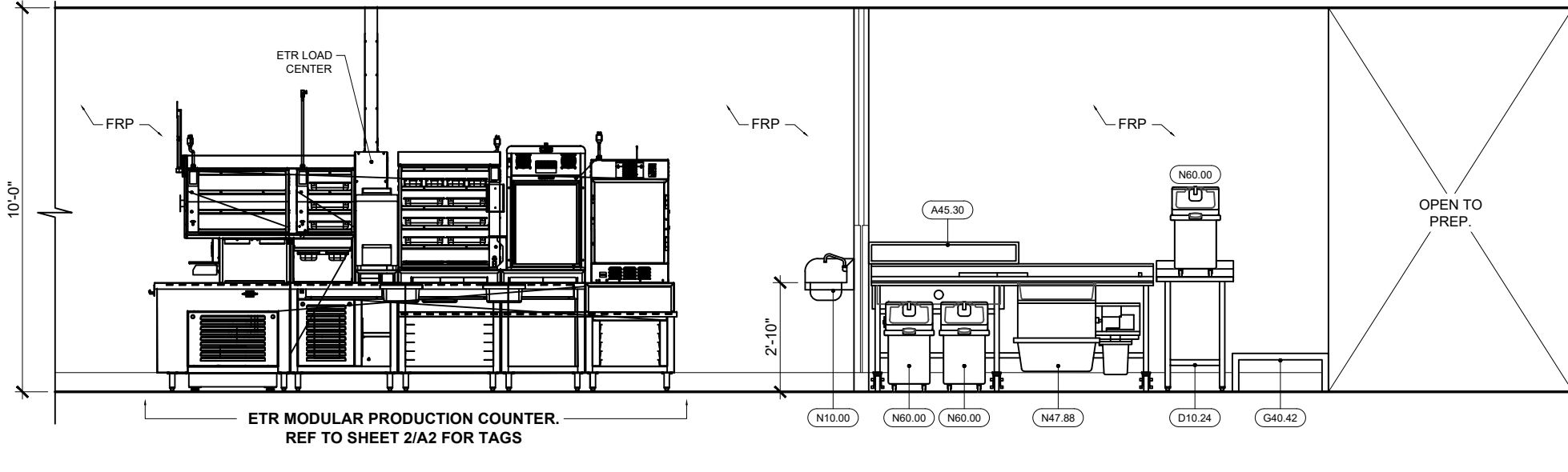
9 PREP AREA A9.1 SCALE: 1/4" = 1'-0"
