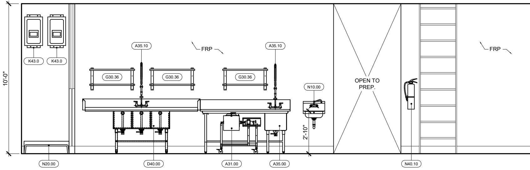
7 WET AREA A9.1 SCALE: 1/4" = 1'-0"
