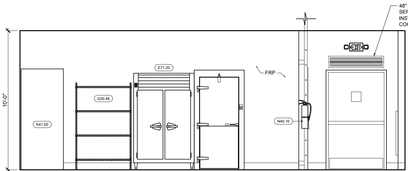
4 PREP AREA A9.1 SCALE: 1/4" = 1'-0"
